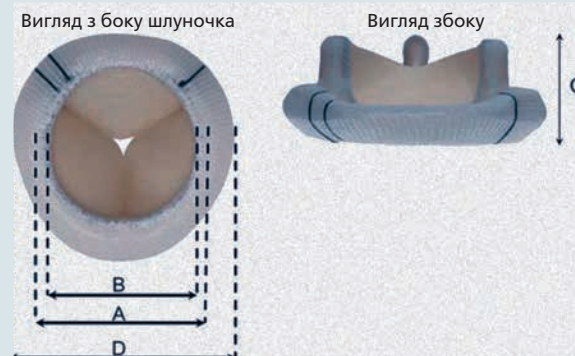
Рис. 6. Розміри стенованого хірургічного біопротеза. Вигляд стенованого біопротеза з боку шлуночка та збоку: (А) зовнішній діаметр базового кільця; (В) внутрішній діаметр базового кільця; (С) висота протеза і (D) зовнішній діаметр шовного кільця [26]
